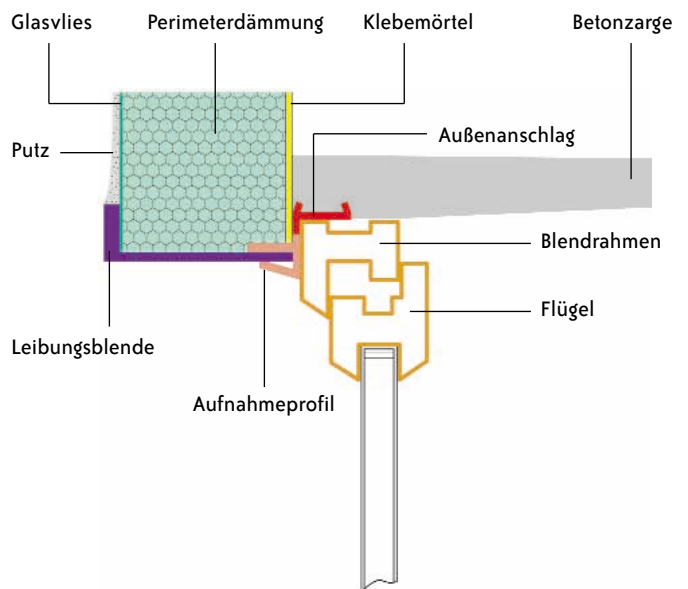
UNIFIX KOMBI-Kellerfenster mit vollständiger Perimeterdämmung und Dämmstoffformteilen für Lichtschacht-Einhängekonsolen
