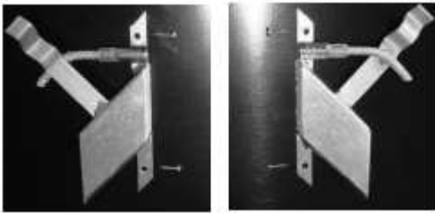
Abbildung 1 und 2 2 Ankerhülsen Typ D und 4 Spaxschrauben in Lieferung enthalten
