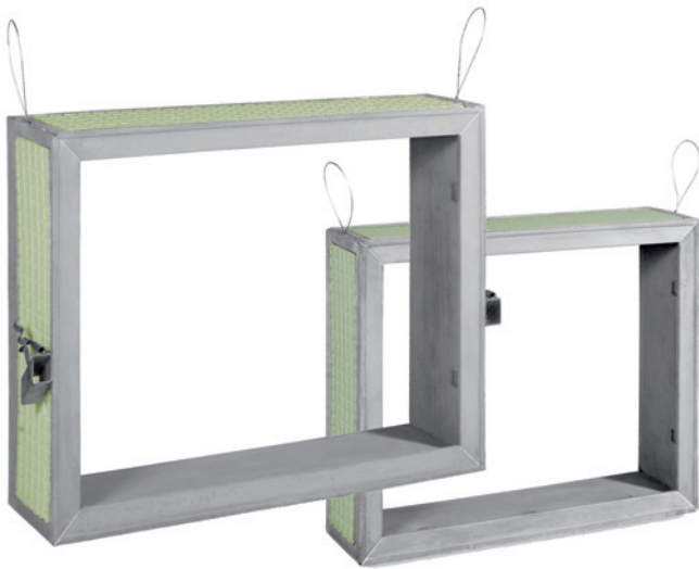
GFB-PROFI mit Kerndämmung und Lichtschachtaufhängung
